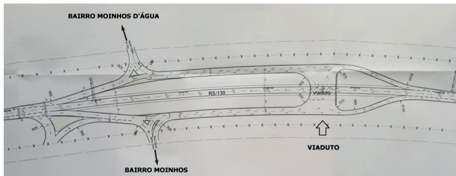
Projeto básico de engenharia de viaduto entre Moinhos e Moinhos d'Água
