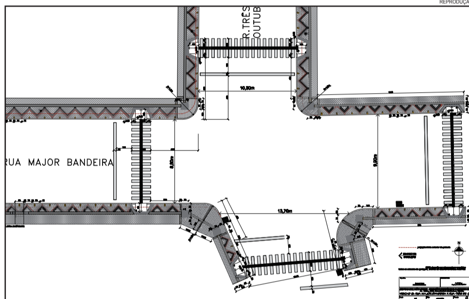
Perspectiva da nova calçada na esquina das ruas Major Bandeira e 03 de Outubro
