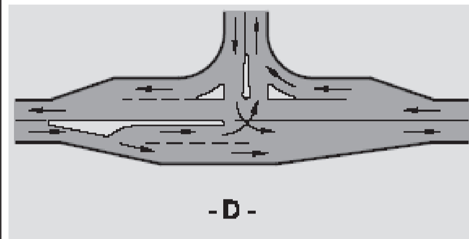
Figura 63 - Interseções de três ramos (T)
