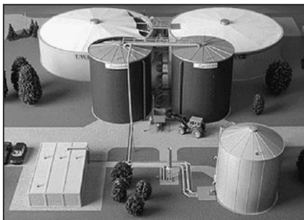
Maquete de uma planta de usina de Biogás projetada por uma empresa asiática
