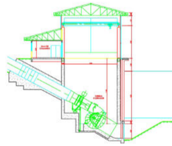
Casa de Máquinas Hidrelétrica Rastro de Auto
